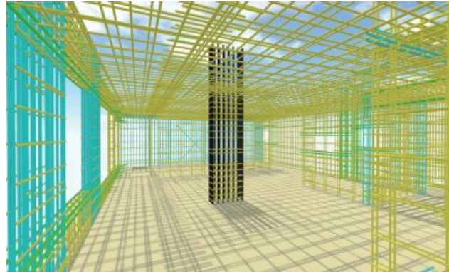
&lt;그림3&gt; 빌더허브의 철근 상세설계 BIM
