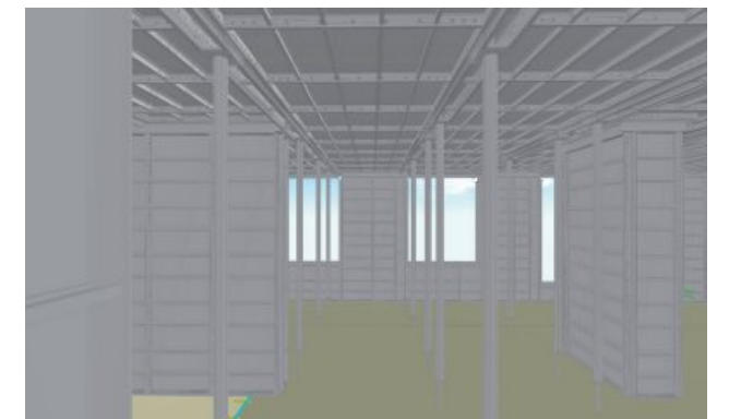
<그림 2> 빌더허브의 거푸집 상세설계 BIM
